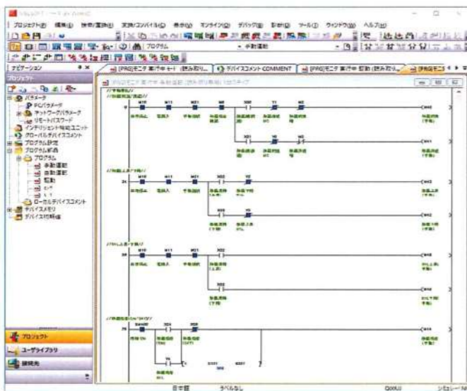
ラダー図
