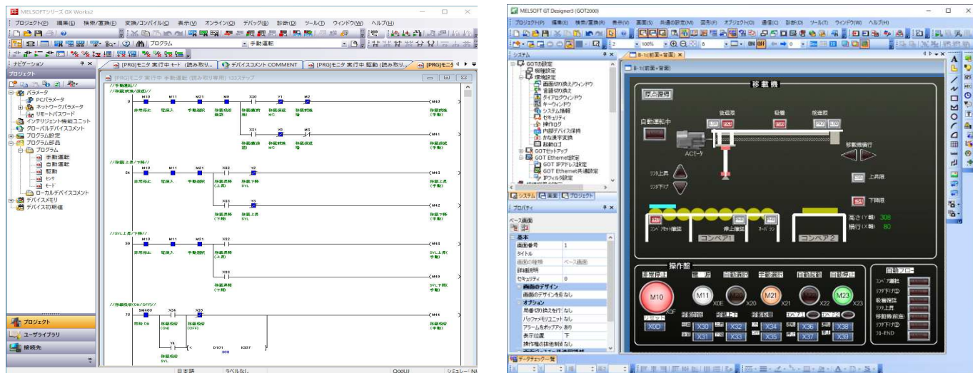
ラダー図
